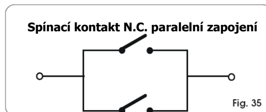
obr. 35 zapojení dvou ovládnání pro OPEN A, OPEN B
